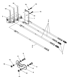
ETB-010481, Zespół trójdrogowy
