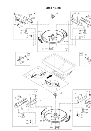
ETB-010452, Tarcza rozsiewająca OMT 10-28
