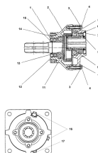
ETB-010465, Specjalna przekładnia nasadowa
