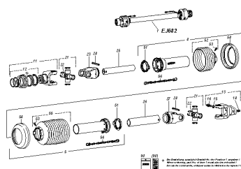
ETB-0000005708, Wałek przegubowo-teleskopowy EJ682 - W 100 E 810 mm, 1 3/8 cala, 6 sztuk
