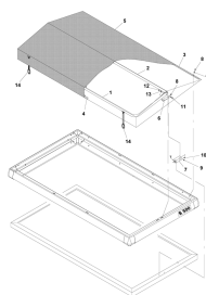
ETB-010485, Składana plandeka S
