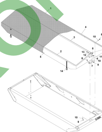
ETB-010486, Składana plandeka L
