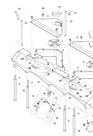
ETB-010491, Lejek środkowy do urządzenia rozsywającego R4, R6, R8
