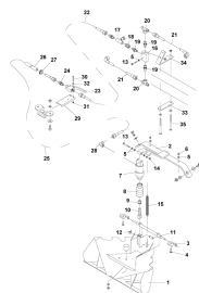
ETB-010458, Ekran rozsiewu granicznego z obu str. z hydraulicznym zdalnym sterowaniem
