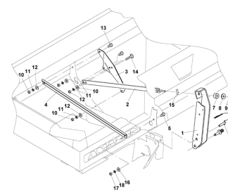
ETB-010501, Wzmocnienie górnej dźwigni zaczepu
