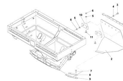
ETB-010487, Osłona przeciwbłotna
