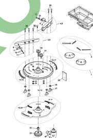
ETB-010450, Tarcza rozsiewająca OS 30-36 / HP
