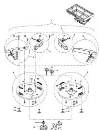
ETB-010448, Tarcza rozsiewająca OS 10-18 / HP
