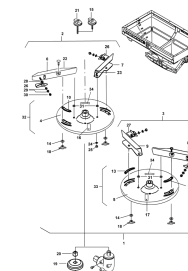
ETB-010447, Tarcza rozsiewająca OS 10-12
