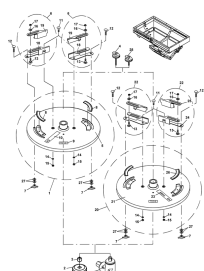
ETB-010453, Tarcza do rozszerzenia granicznego TS 5-9
