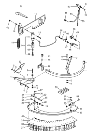
ETB-010459, Rozpierzacz obramowania, lewy "Limiter M"
