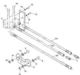
ETB-010480, Zespół dwudrogowy
