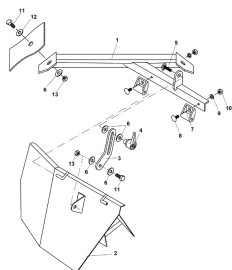
ETB-010457, Ekran rozsiewu granicznego mechaniczny
