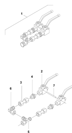
ETB-010482, Łącznik zasuwy
