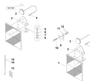
ETB-010490, Oświetlenie przednie
