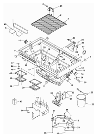
ETB-010444, Rama ze zbiornikiem
