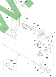
ETB-010466, Wałek mieszadła i jarzmo łańcucha
