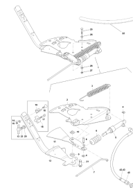
ETB-010467, Dno z otworami mechaniczne
