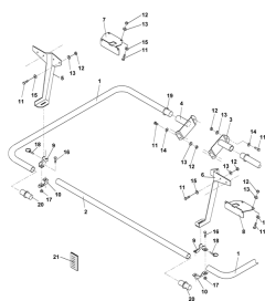
ETB-010461, Rurowy pałąk ochronny odchylany
