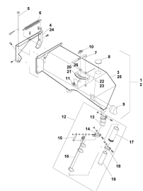
ETB-010493, Lejek odchylany do urządzenia rozsiewającego R8
