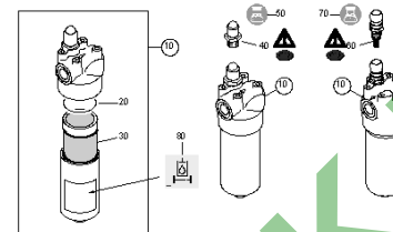
ETB-006791, Filtr hydrauliczny ciśnieniowy
