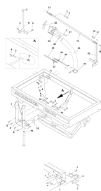
ETB-010499, Zestaw montażowy do żmijki załadunkowej
