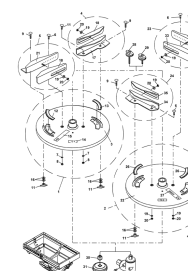
ETB-010456, Tarcza do rozszerzenia granicznego TS 4
