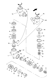
ETB-010464, Przekładnia kątowna
