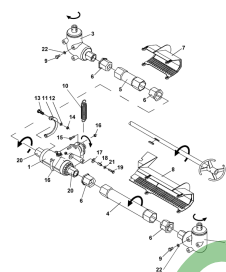
ETB-010462, Napęd ZA-M
