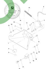
ETB-010497, Urządzenie do ustawiania odpowiedniej dawki rozsiewu
