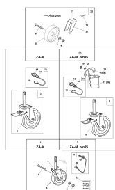
ETB-010488, Kółka transportowe do ZA, hamowane
