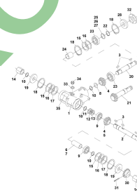
ETB-010463, Przekładnia wejściowa i specjalna przekładnia wejściowa
