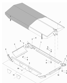
ETB-010484, Nadstawka nad zbiornik L 1000
