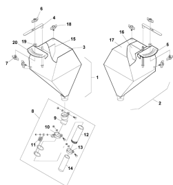
ETB-010492, Lejek zewnętrzny do urządzenia rozsiewającego
